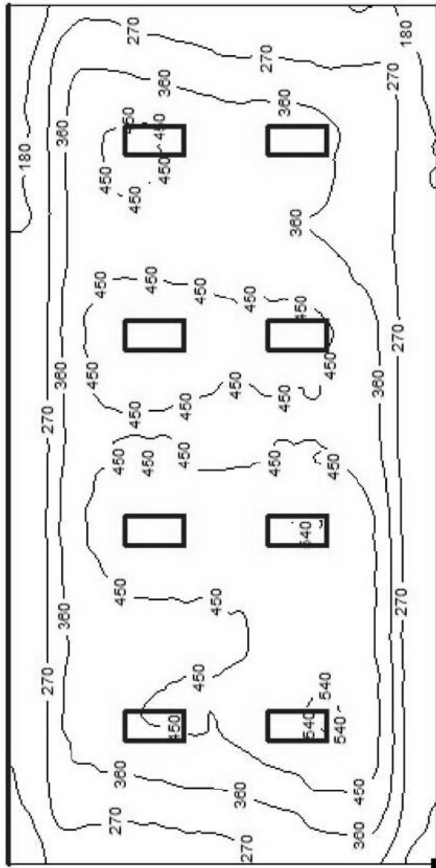
BELICHTUNGSSITUATION SPORTHALLE
